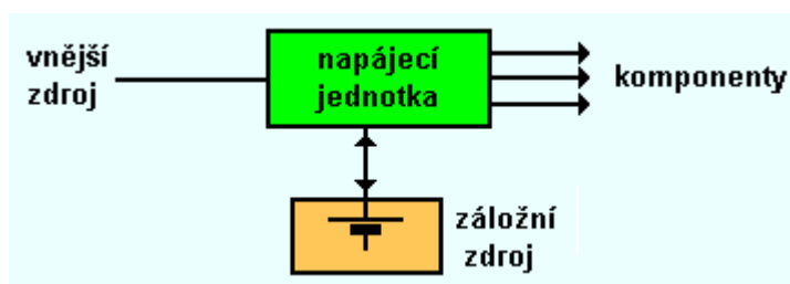
Obr.22 Schéma zdroje typu A
