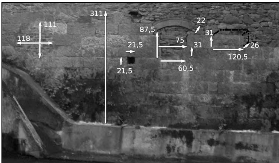
Obr. 1a. Naměřené hodnoty dílců základové jednotky (autor)
